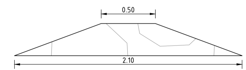
Principeprofiel 3-3: Drempel (midden) schaal: 1:20
