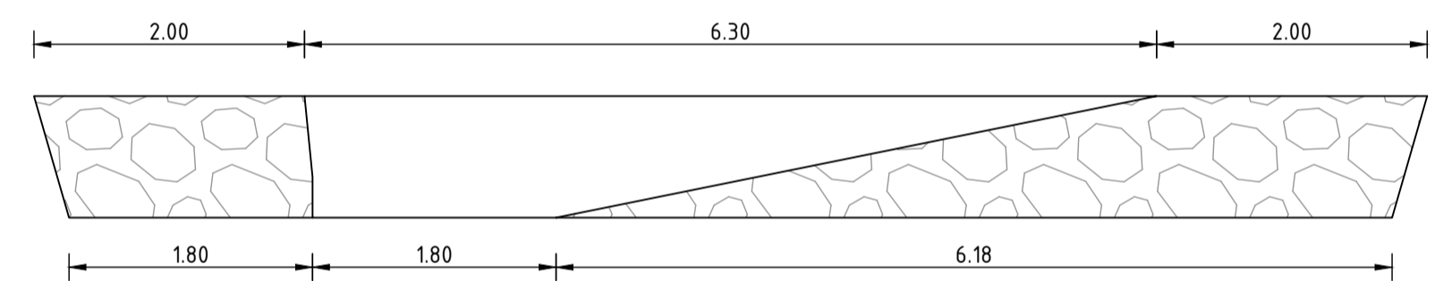
Principeprofiel 1-1: Doorsnede drempel schaal: 1:20
