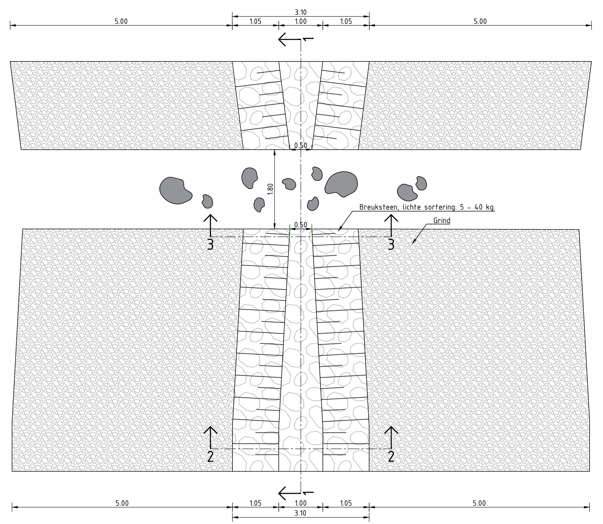
Detail 1: Bovenaanzicht drempel nevengeul schaal: 1:50
