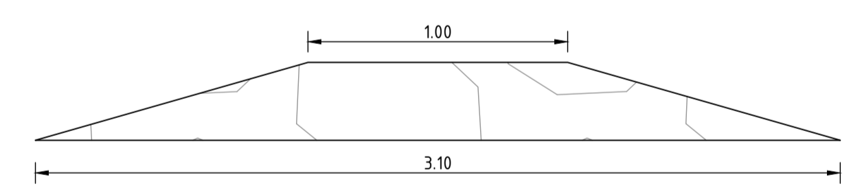
Principeprofiel 2-2: Drempel (zuid zijde) schaal: 1:20
